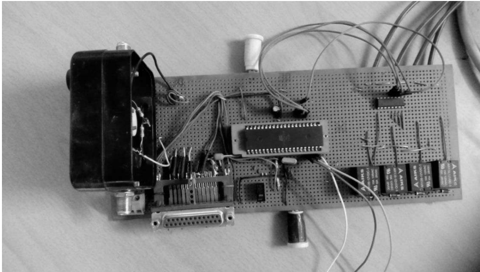
الشكل (4-14) الدائرة الإلكترونية للنظام
