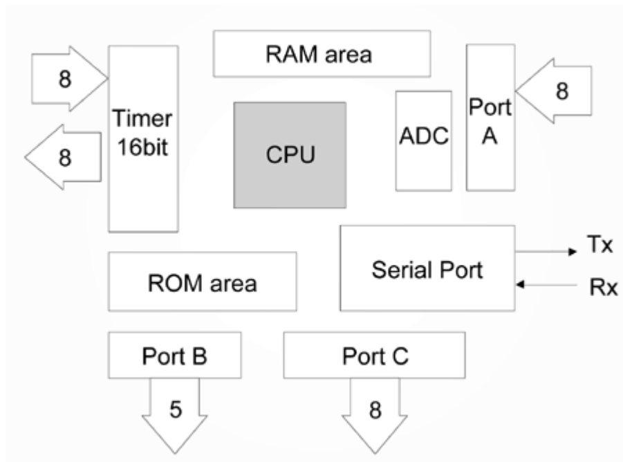
الشكل (15-3) المخطط الصندوقي للتحكم (Atmega32A)
