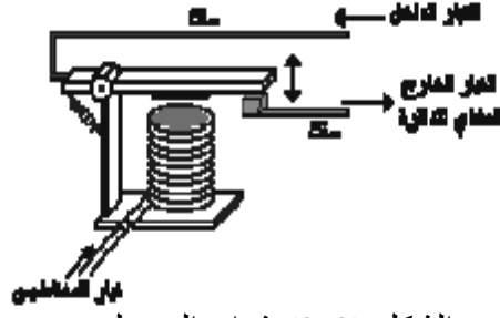
الشكل (3-9) ذراع المرحل
