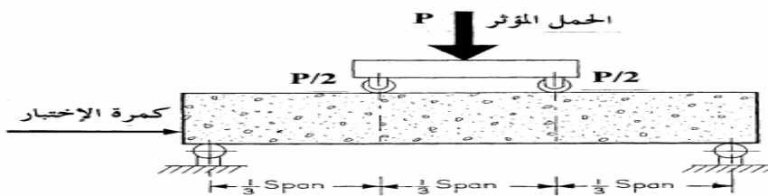
شكل الكمرة في مقاومة الانحناء
