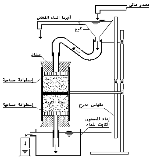
شكل رقم (٦-٢) جهاز ضغط الماء الثابت لقياس نفاذية التربة الرملية والحصوية
