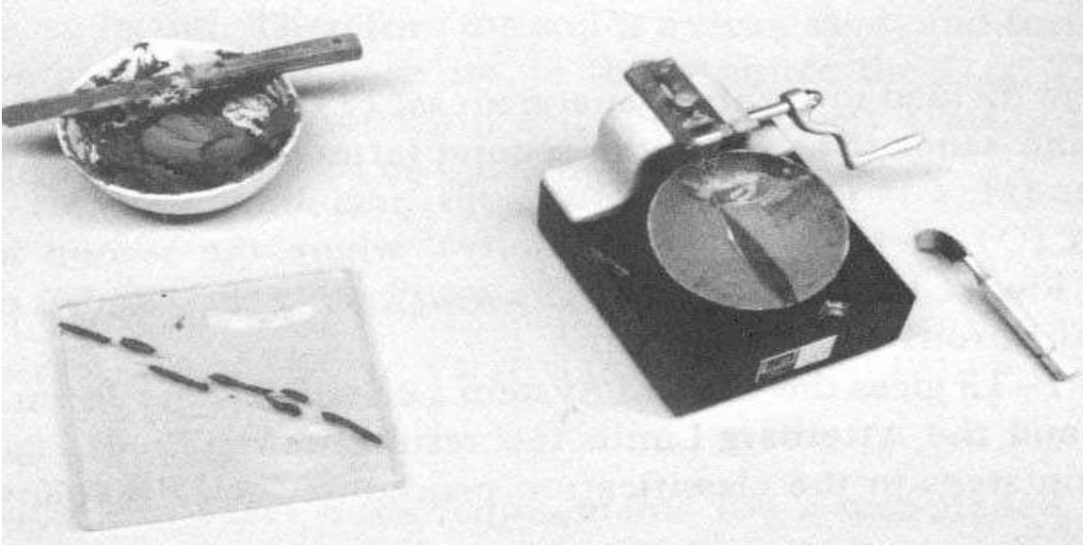
شكل رقم (١-٢) يوضح: جهاز كازجراند - أداء التحزير
