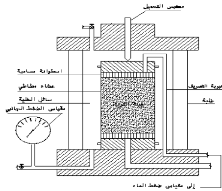
شكل رقم (٨-٢) توضيح: جهاز الانضغاط ثلاثي المحاور
