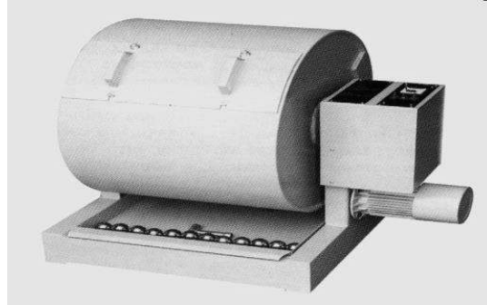
شكل رقم (٢-٤) جهاز لوس أنجلوس
