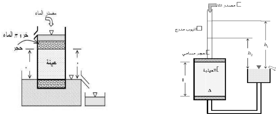
شكل رقم (٥-٢) يوضح: جهاز ضغط الماء المتغير
