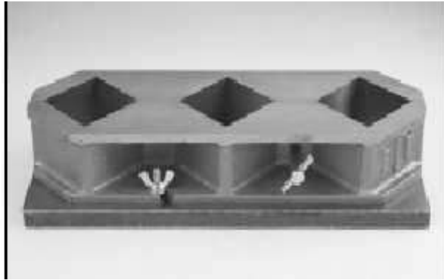
مجموعة من ثلاث قوالب مكعبة للمونة
