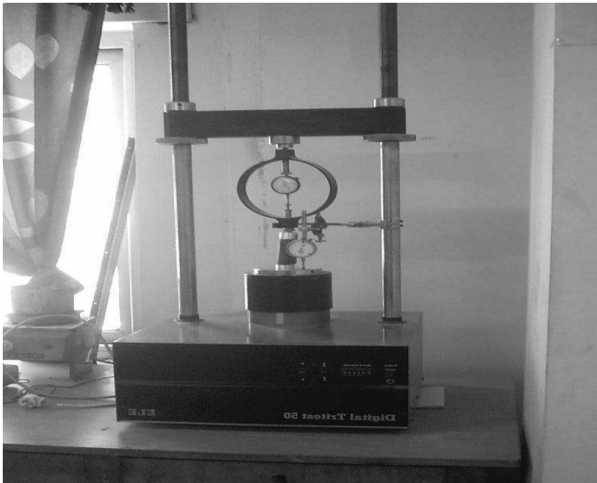
شكل رقم (٩-٢) توضيح: جهاز التحميل
