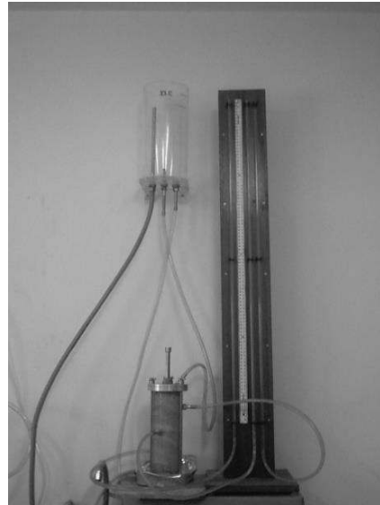
شكل رقم (٦-٢) جهاز ضغط الماء الثابت لقياس نفاذية التربة الرملية والحصوية
