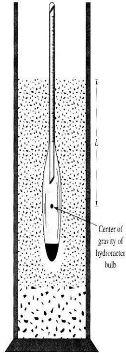
شكل رقم (٢-٣) توضيح: جهاز الهيدرومتر
