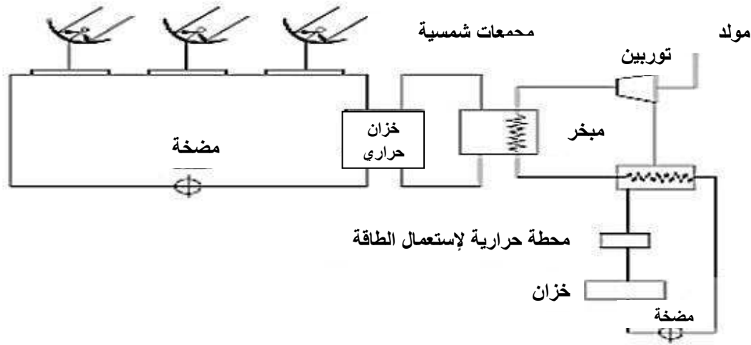
الشكل (1-3) يوضح محطة توليد الطاقة الكهربائية بالتحويل الحراري للطاقة الشمسية
