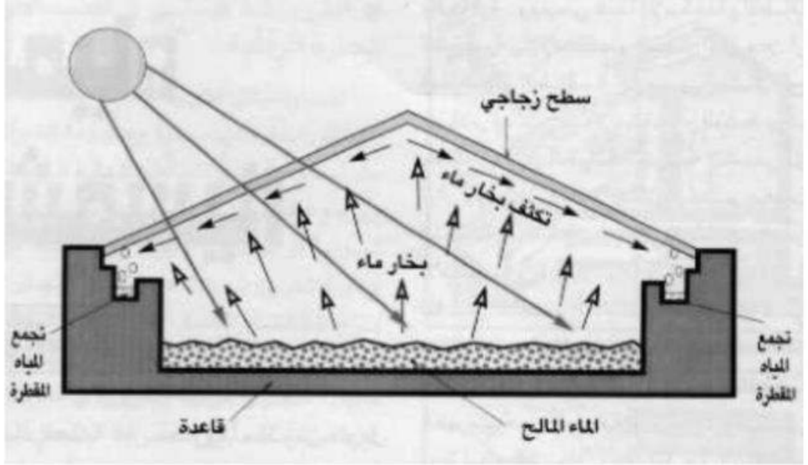
مخطط (3-5) مبسط للمقطرات الشمسية الحرارية
