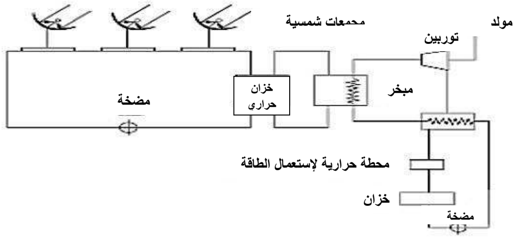
الشكل (1-3) يوضح محطة توليد الطاقة الكهربائية بالتحويل الحراري للطاقة الشمسية
