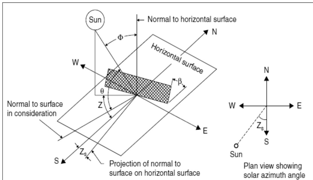
الشكل (4-1): الزوايا الشمسية
