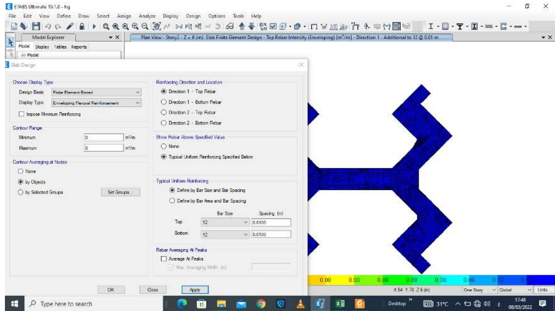
الشكل (4-21) يوضح حديد التسليح العلوي في اتجاه X لبلاطة الطابق الثاني.
