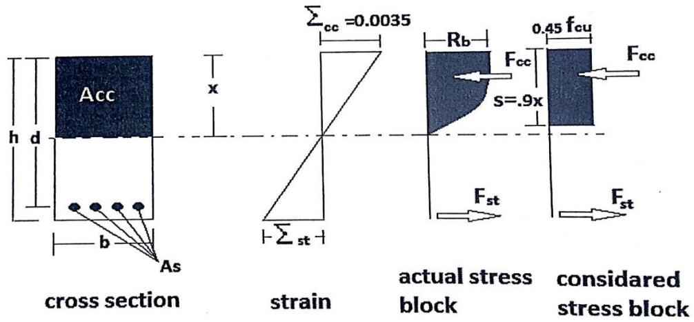
شكل (2-6) مخطط الإجهادات والتشوهات وفق طريقة حالة الحدود القصوى لمقطع مستطيل
