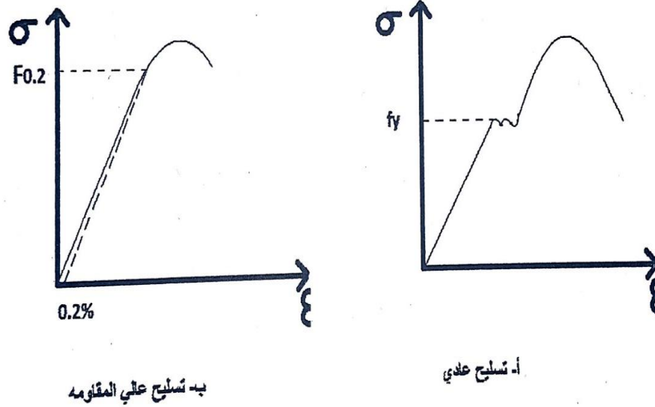
شكل (2-7) العلاقة بين الإجهادات والتشوهات لفولاذ التسليح
