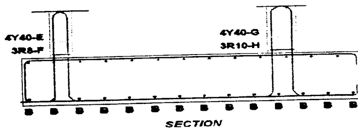
شكل (4-2-4) يوضح حديد تسليح القاعدة المشتركة
